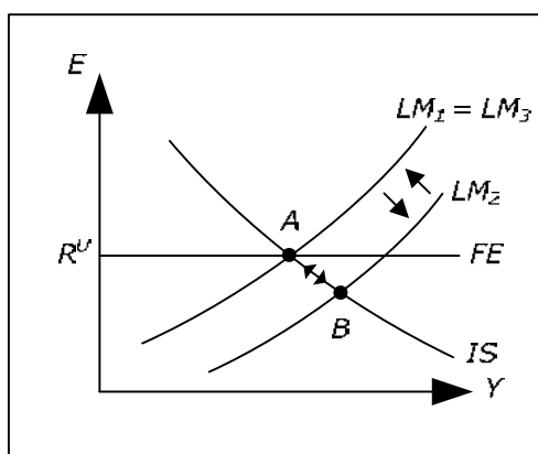
Fig. 16.3: IS-LM-FE.
